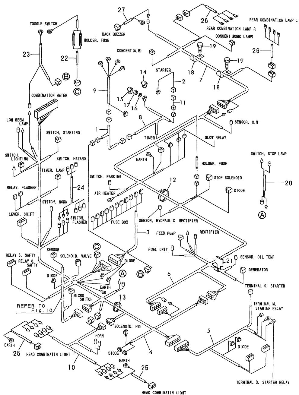
Fig. 11 WIRING
