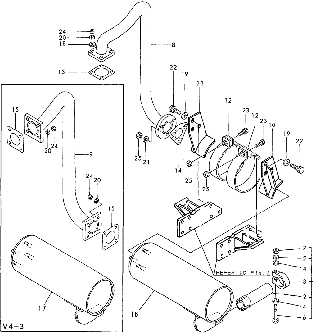
Fig.4 SILENCER
