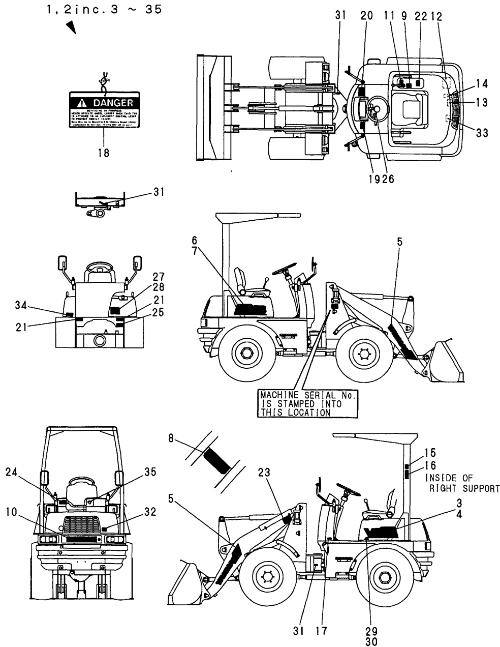
Fig.1 LABEL
