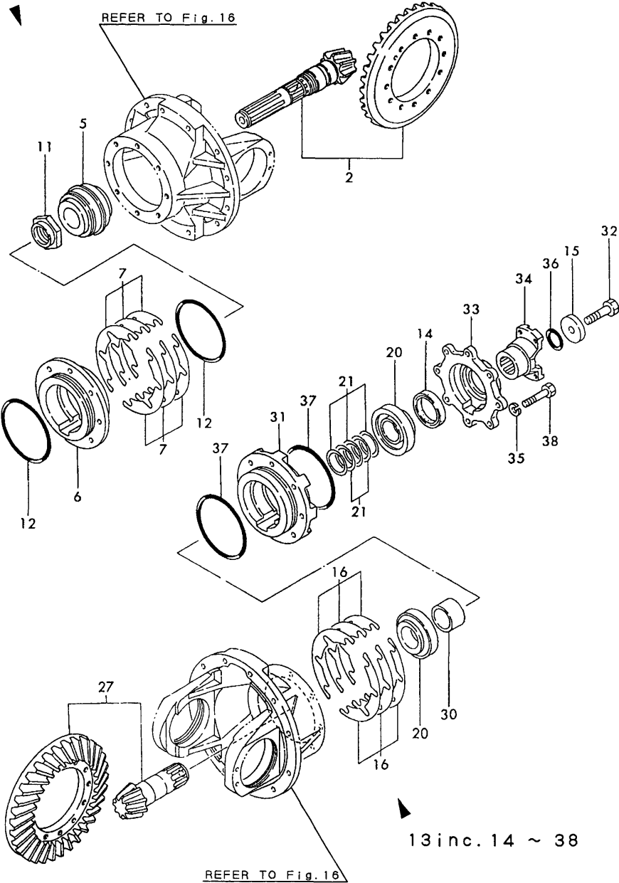
Fig.14 SPIRAL BEVEL GEAR (V3-3) 1 inc. 2 ~ 12
