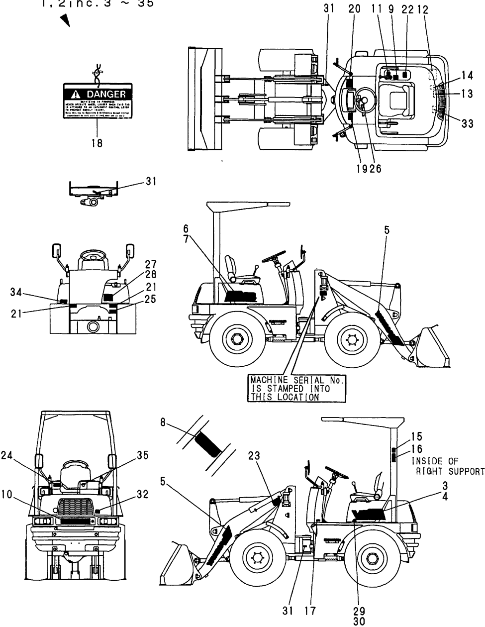
Fig.1 LABEL
