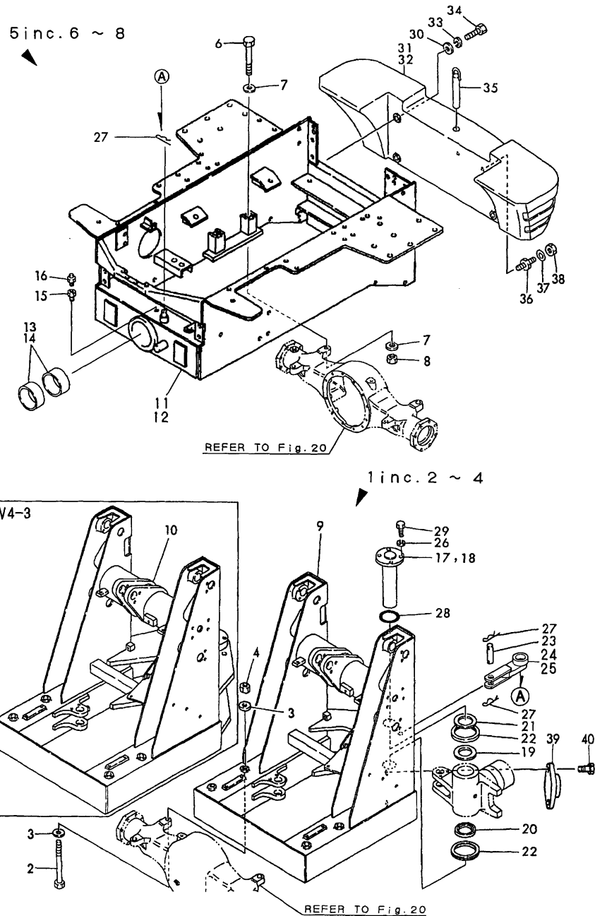
Fig.31 FRAME
